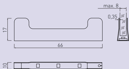
Wymiary klipu
